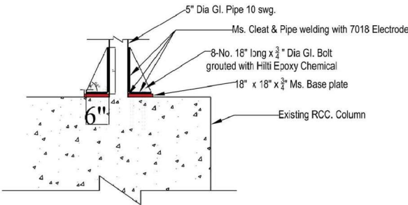
Typ. Section. A-A
